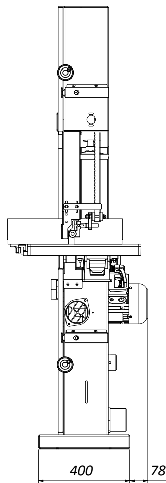
Seitenansicht:
