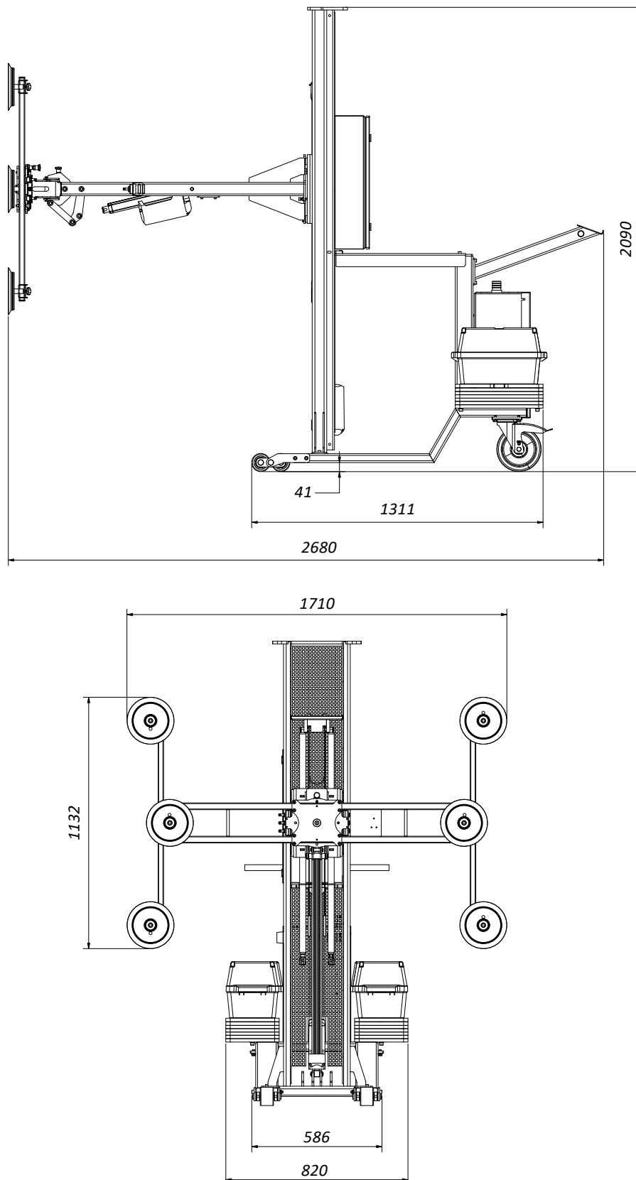
Abbildung 3: Abmessungen ML-120
