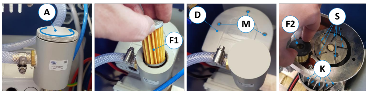
Abbildung 24: Vakuumpumpe mit Filtereinsätzen und Kohleschiebern
