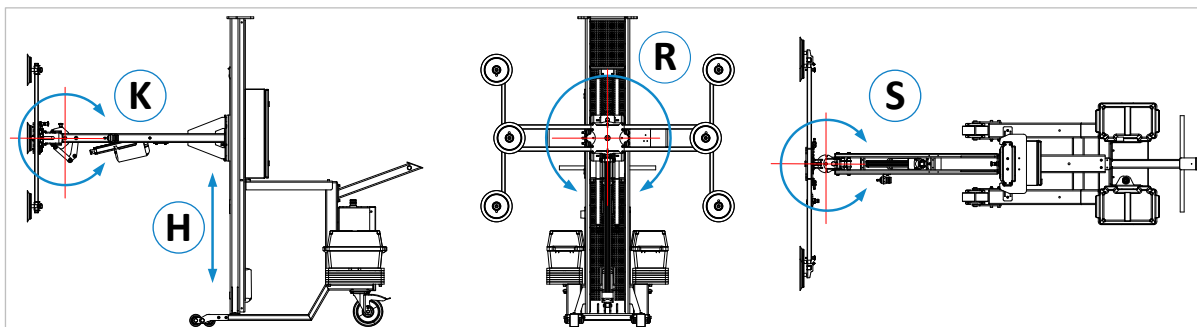
Abbildung 8: Verstellmöglichkeiten ML-120
