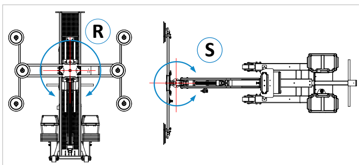
Abbildung 12: Rotations- und Schwenkverstellung
