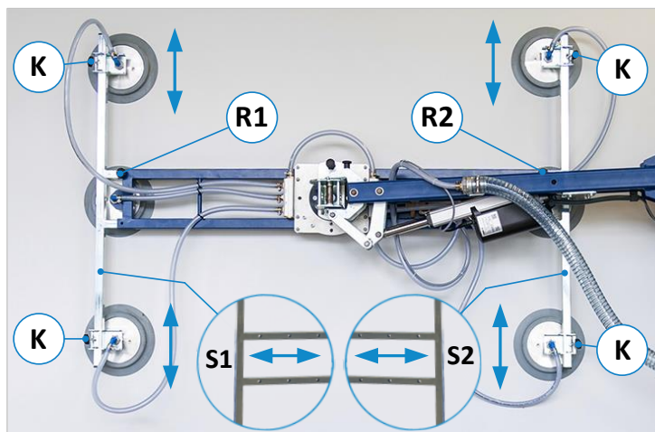
Abbildung 20: Verstellung der Sauggreifer-Positionen
