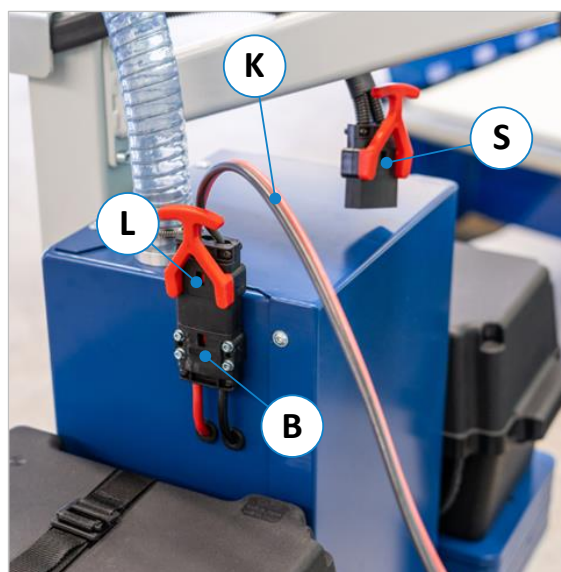
Abbildung 23: Ladekabel im eingesteckten Zustand
