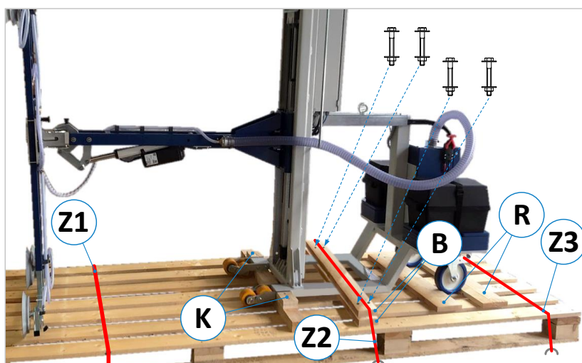
Abbildung 5: Mobillifter auf Palette sichern
