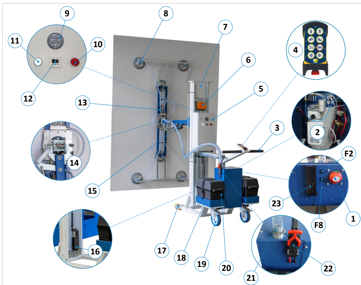
Abbildung 6: Komponenten und Bedienelemente ML-120
