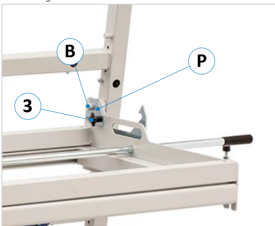
Abbildung 6: Schwenkrahmen demontieren
