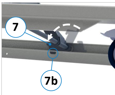
Abbildung 17: Sicherungs-Sperrklinge
