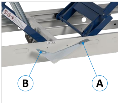
Figure 6 : étrier de pied et frein
