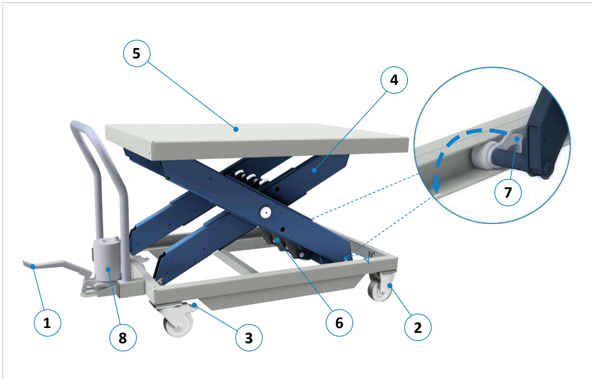
Figure 3 : composants et éléments de commande HS 2000 | FH
