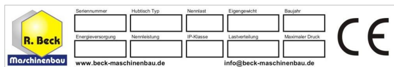
Abbildung 2: Typenschild
