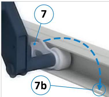
Figure 9 : cliquet d'arrêt
