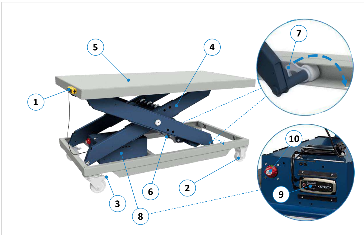
Figure 4 : composants et éléments de commande HS 2000 GRANDE | AH
