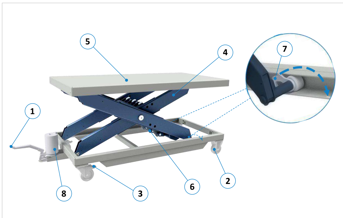
Figure 3 : composants et éléments de commande HS 2000 GRANDE | FH
