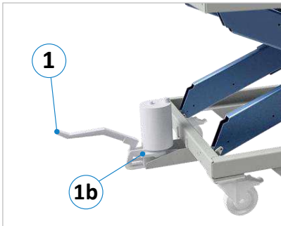
Figure 6 : pédales de réglage
