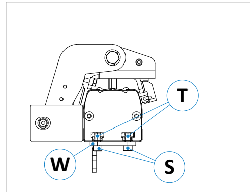
Figure 3 : vue latérale de l'unité montée
